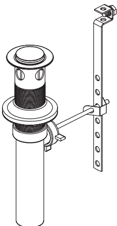
RP38958▲ Pop-Up with Metal Flange and Plastic Tail Piece Less Lift Rod Drenaje automático con brida de metal y la pieza de cola plástica menos la barra de alzar Renvoi mécanique avec collerette en métal et raccord droit de vidange en plastique sans la tige de manoeuvre
